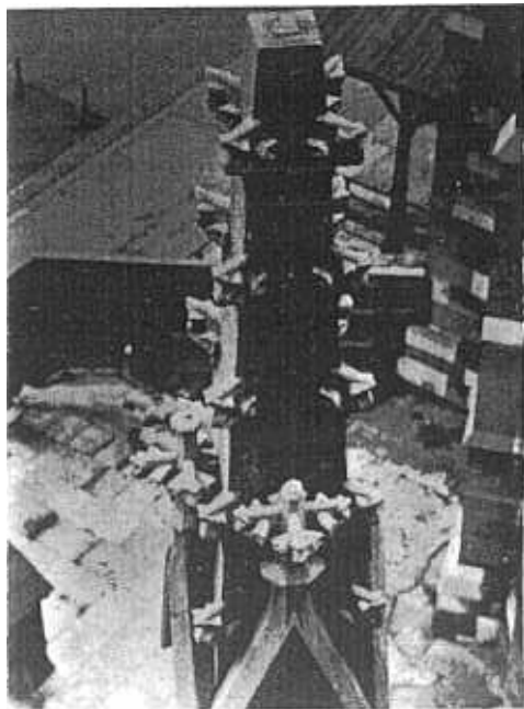
Fig. 44 Vienne, Votivkirche. Tenon de pierre arraché par manque de résistance à la traction.
