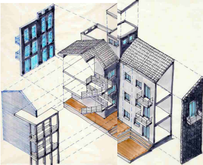
Axonometric, "Rehabilitation of House Callejón del Chicheme", 4 th St. Casco Antiguo. Pmá. 2002.
